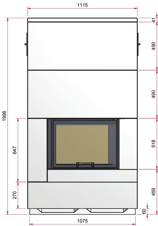
Frontansicht M 1:20
