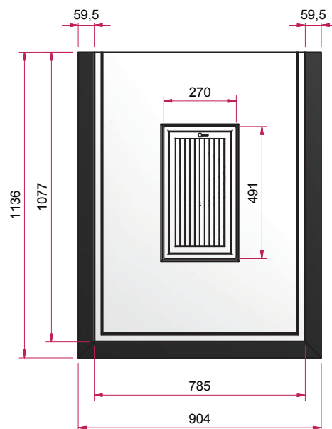
Draufsicht M 1:20
