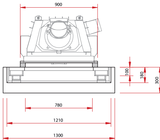
Draufsicht M 1:25
