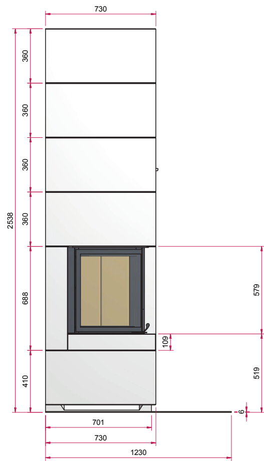
Seitenansicht M 1:25
