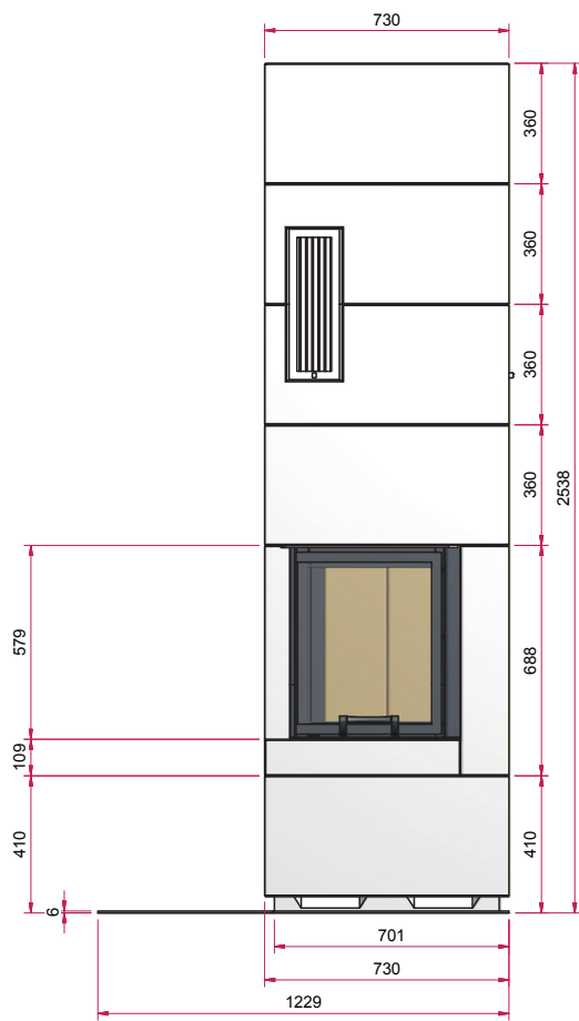
Frontansicht M 1:25
