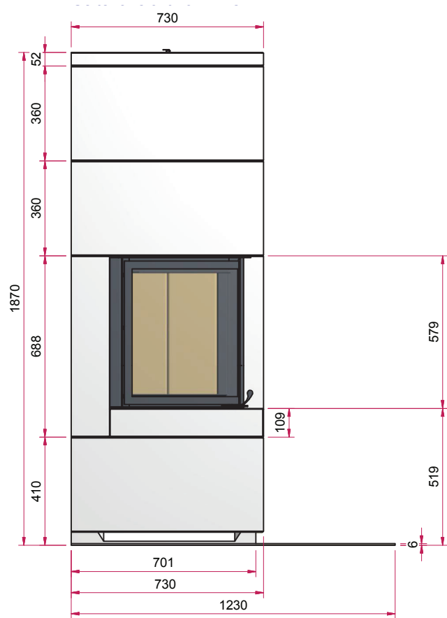
Seitenansicht M 1:20
