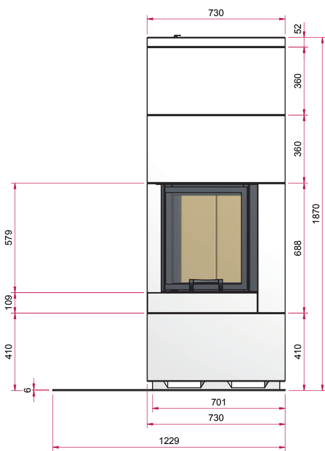
Frontansicht M 1:20
