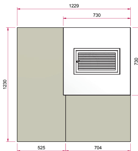
Draufsicht M 1:20
